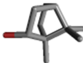
Borneol
